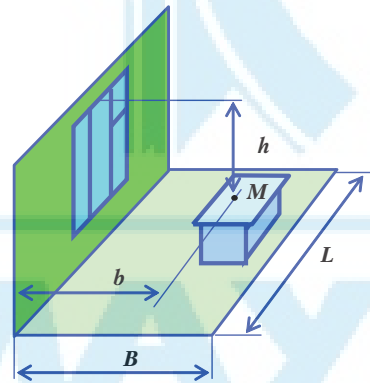
Рис. 3. До визначення світлової характеристики вікон
