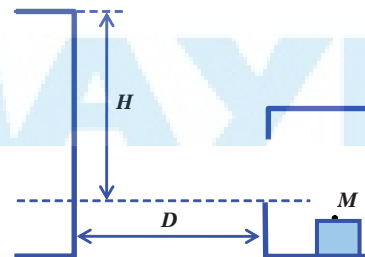
Рис. 4. Затінення вікон будівлею, розташованою напроти
