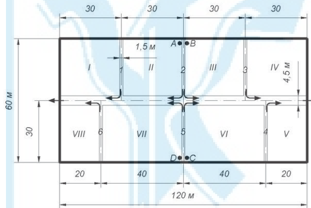
Рис. 1. Загальний схематичний план цеху
