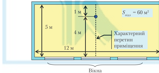
Рис. 5. Ескіз приміщення: М – розрахункова точка на робочій поверхні
